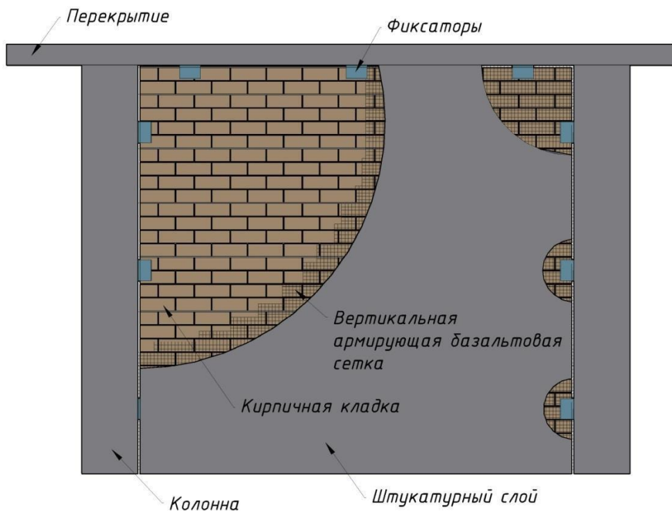
Рисунок П.3.1 - Общий вид перегородки, усиленной вертикальной сеткой СБНПс ГРИДЕКС-К
