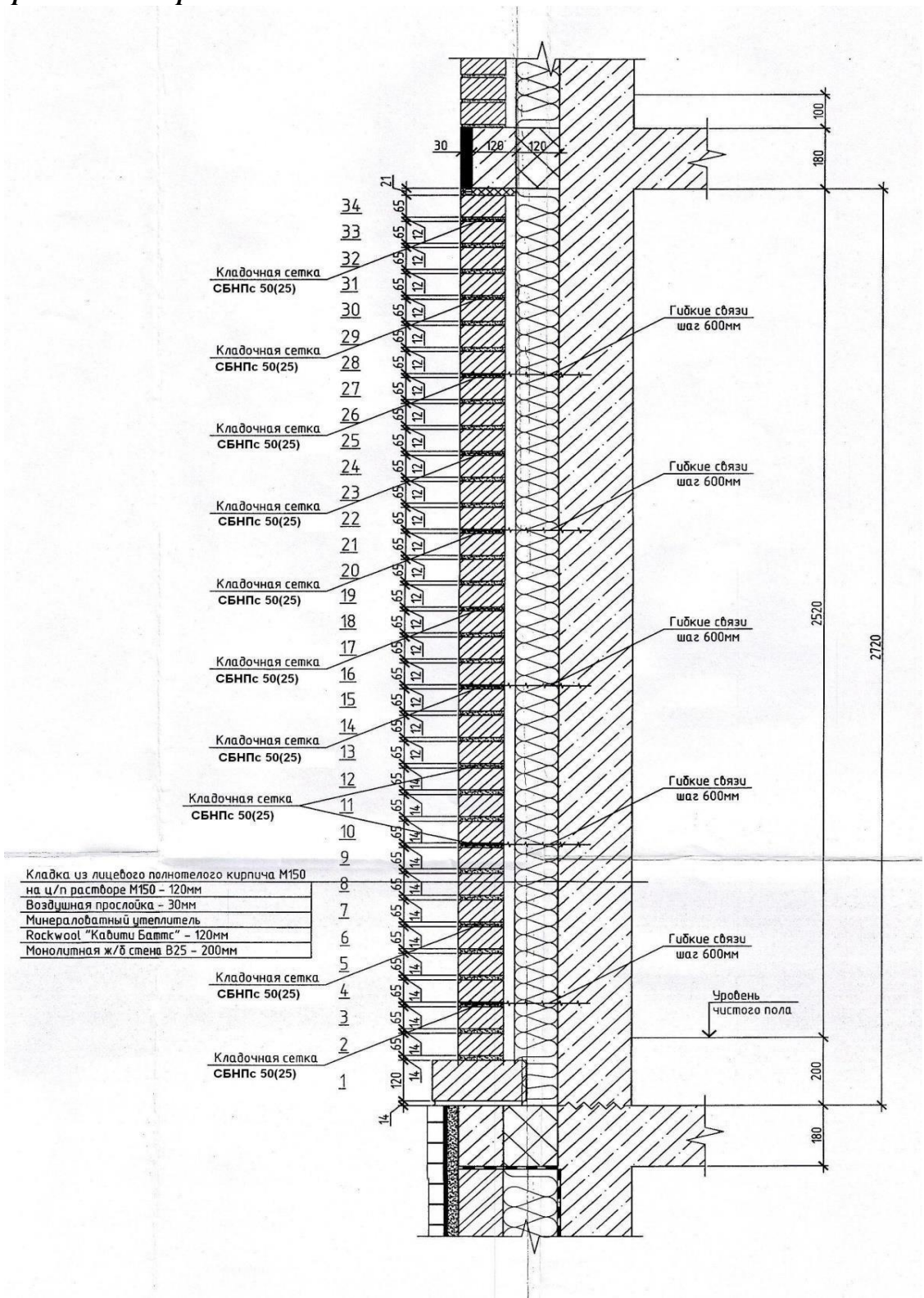
Рисунок П.2.5 Сечение по наружной стене
