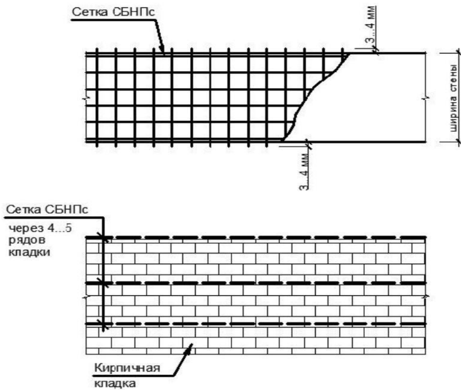
Рисунок 6.2 - Схема армирования кладки сеткой СБНПс ГРИДЕКС-К
