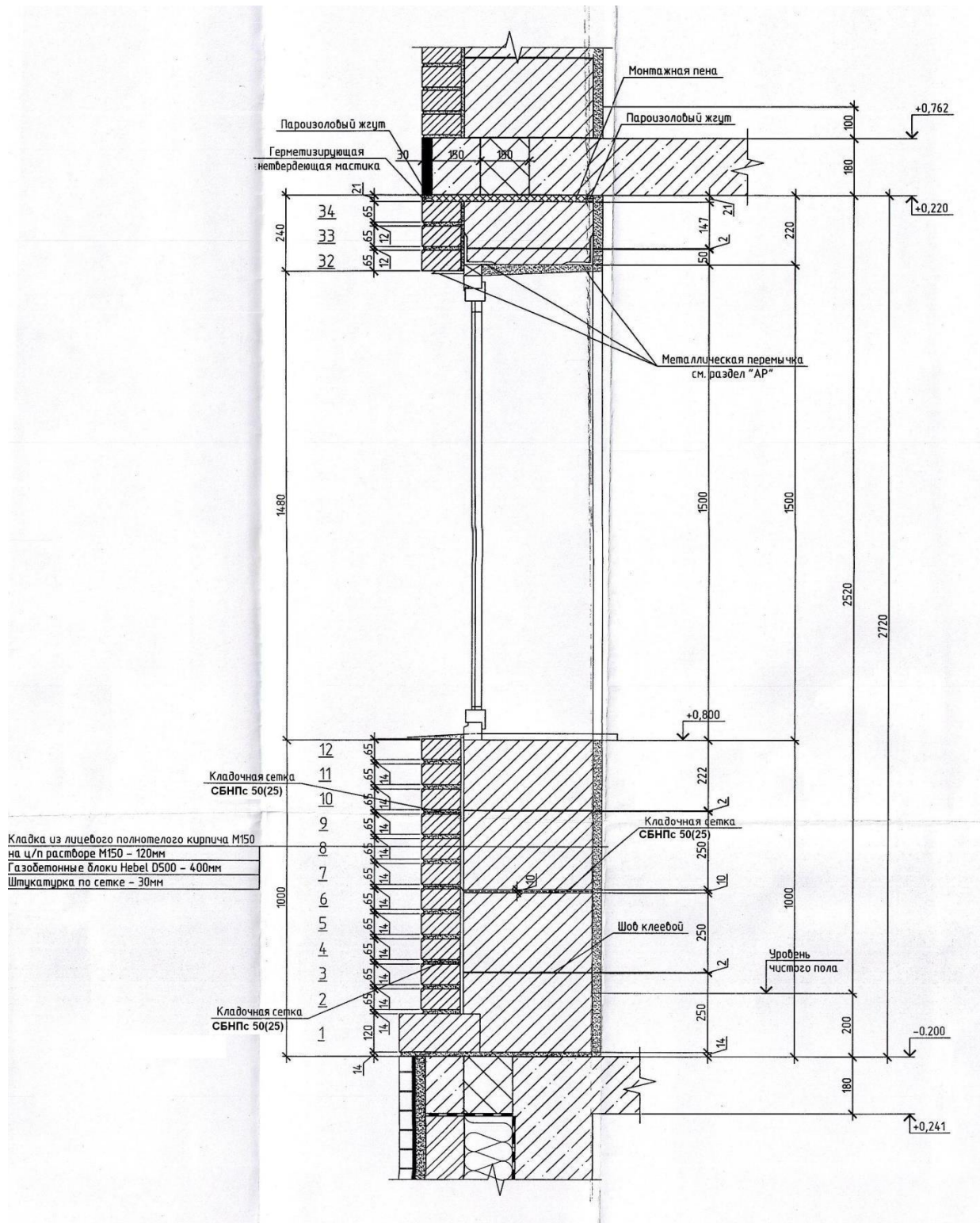
Рисунок П.2.6 Сечение по наружной стене в зоне оконного проема
