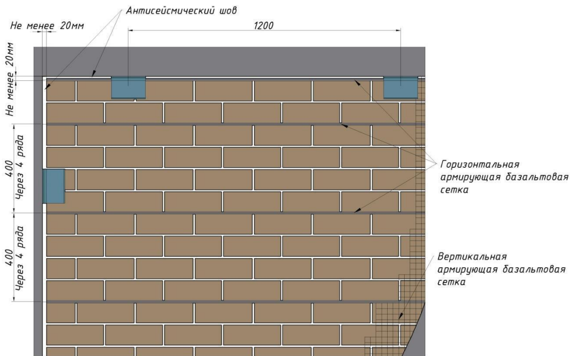
Рисунок П.3.2 - Общий вид перегородки, усиленной базальтовой сеткой СБНПс ГРИДЕКС-К, установленной в горизонтальные швы кладки
